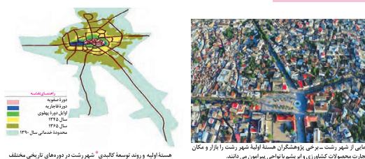
هسته اولیه و روند توسعه کابردی شهرنشست در دوره‌های تاریخی مختلف
